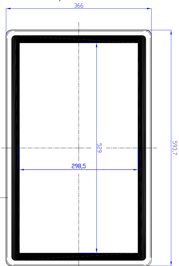
FRONTANSICHT
